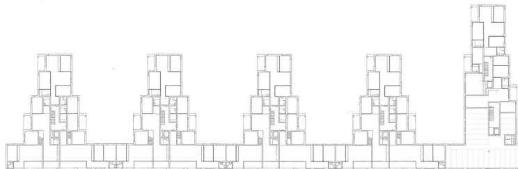
2. Obergeschoss
